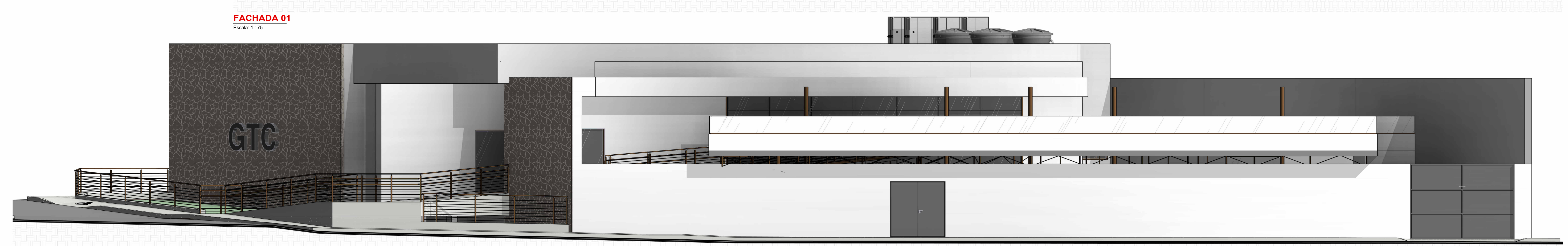
FACHADA 01 Escala: 1:75
